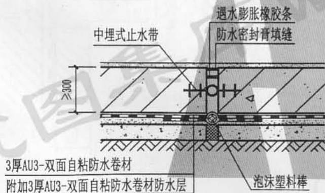
② 底板变形缝
