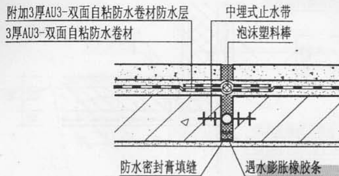
① 顶板变形缝
