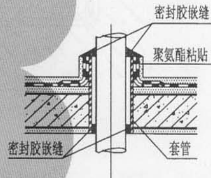
⑤ 穿楼板套管
