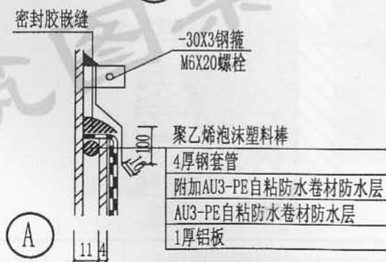
① 铁皮烟囱
