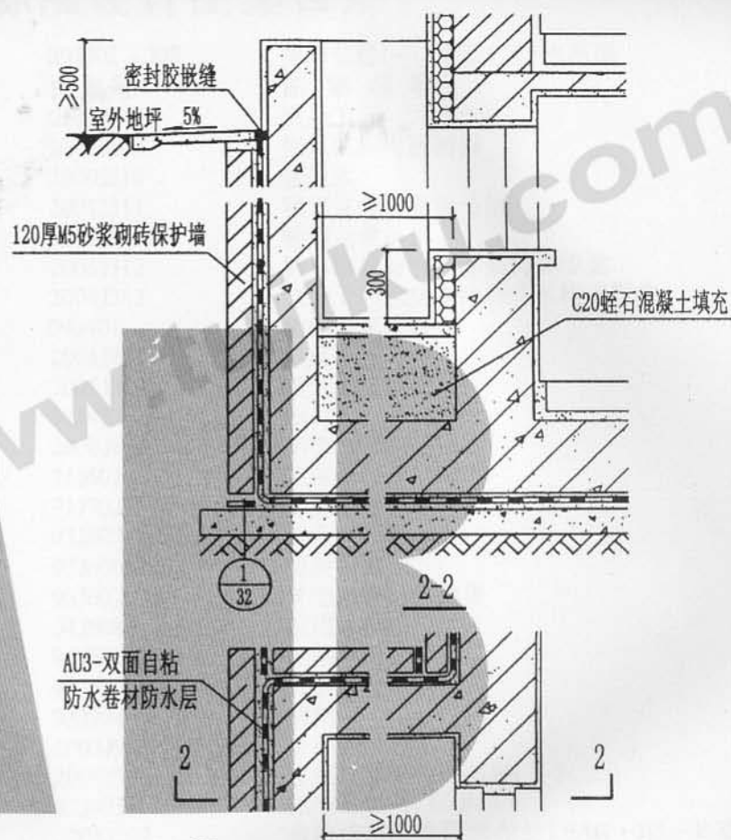
2 窗井平面示意 (二)
